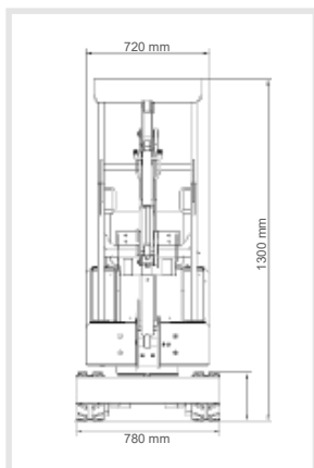
Dimensões principais
